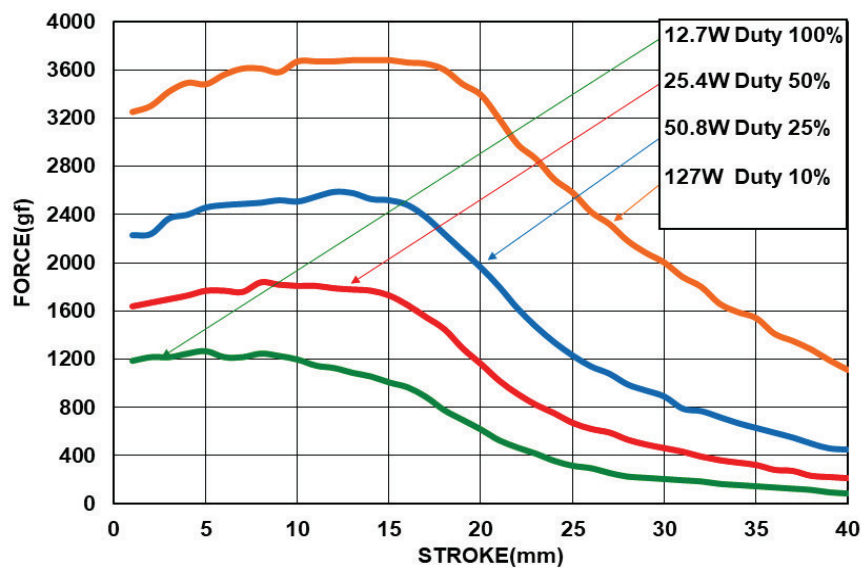
Kraft-Wege-Diagramm / Stroke-Force-Diagram
