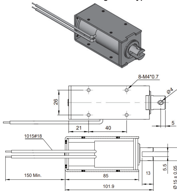
Ziehende Ausführung / Pull Type
